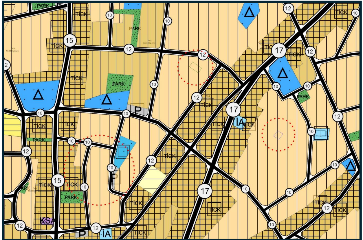
Şekil 2. Yürürlükte Olan Mevcut 1/5000 Ölçekli Nazım İmar Planı
